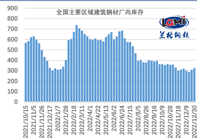
图 15 建材厂内库存(万吨)
