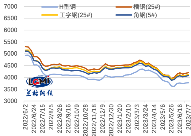
图 5 型材十大城市均价走势（元/吨）
