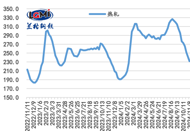
图20 热轧社会库存(万吨)
