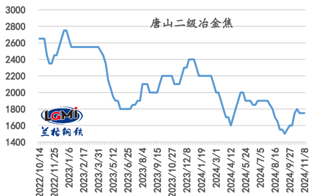
图 29 焦炭价格（元/吨）
